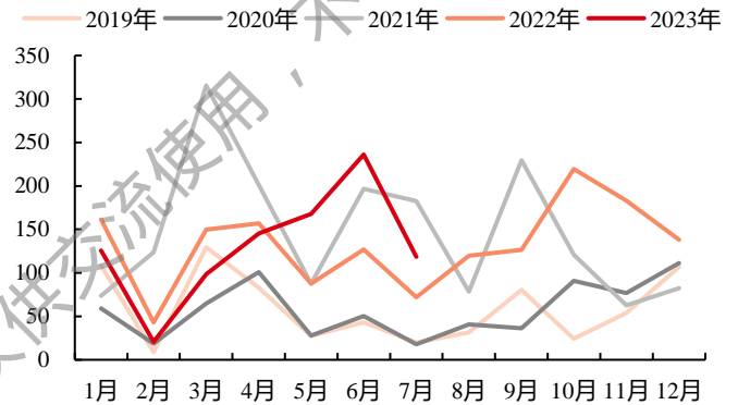
图 22：承接新订单量 | 单位：万载重吨
